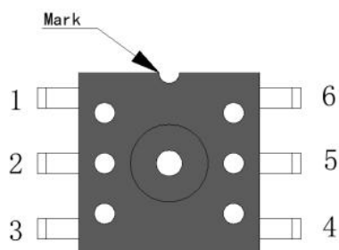
图 1. 引脚示意图
