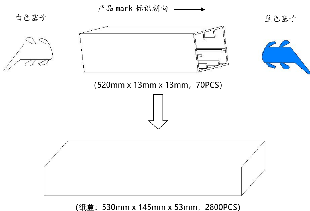
图 10.包装示意图
