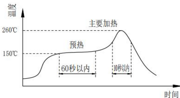
图 8. 回炉温度设置条件
