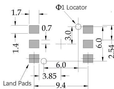
图 7.推荐焊盘尺寸
