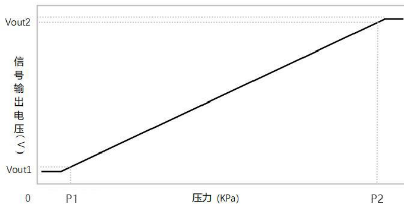
图3 输出曲线
